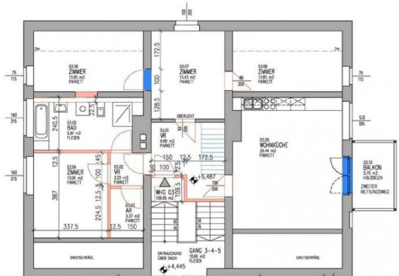
GRUNDRISS OG
